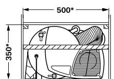
Combi Combi D 6 (E) Afmetingen & gewicht:
