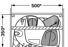
Combi 4 (E) / Combi 6 (E) Afmetingen & gewicht:
