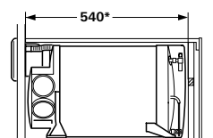
Combi Combi D 6 (E) Afmetingen & gewicht:
